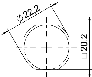
Lochbild
