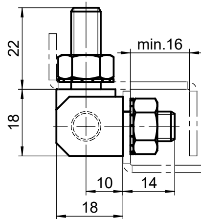
Einbaubeispiel example of installation
